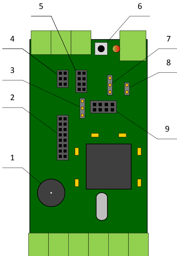
Рисунок 3 – Расположение элементов на плате Устройства
