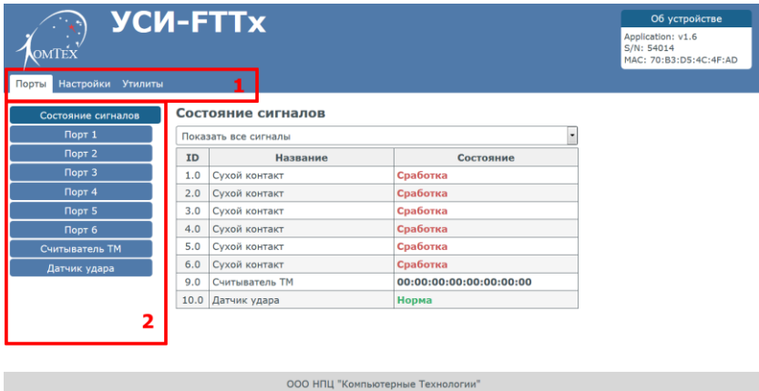
Рисунок 2 – Веб-страница Устройства
