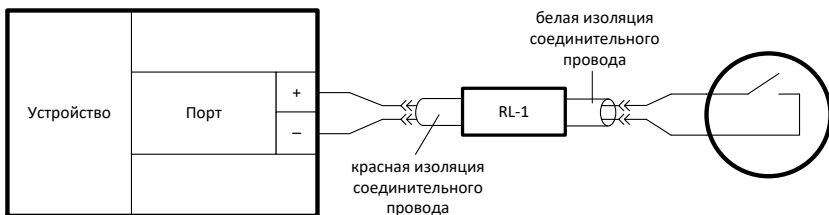
Рисунок 8 – Подключение датчика с помощью модуля RL-1
