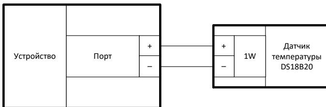
Рисунок 14 – Схема подключения датчика температуры
