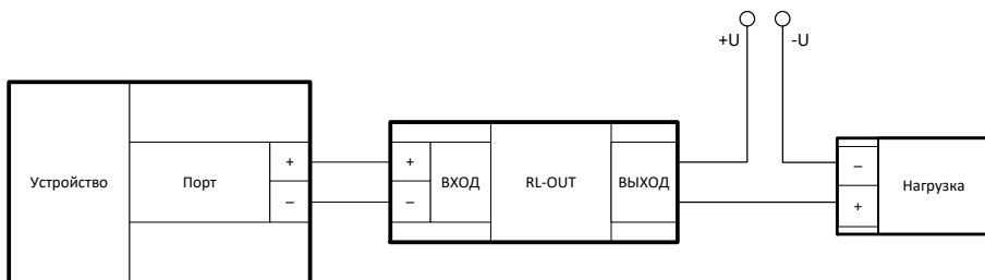
Рисунок 13 – Подключение модуля RL-OUT
