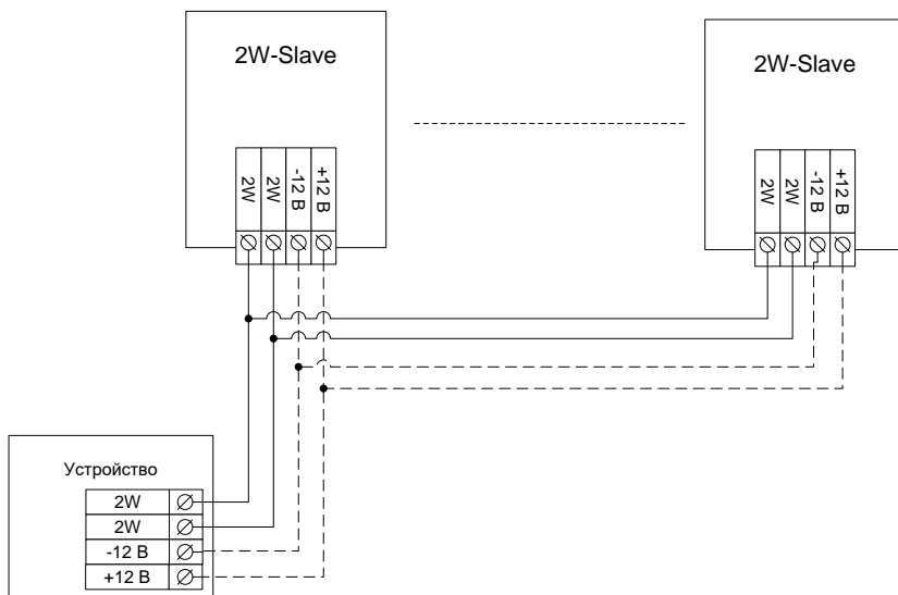
Рисунок 6 – Подключение 2W-slave устройств
