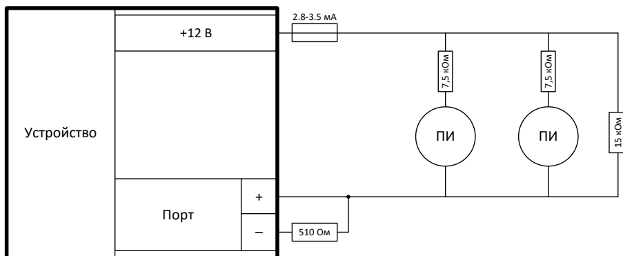
Рисунок 19 – Схема подключения пожарного шлейфа
