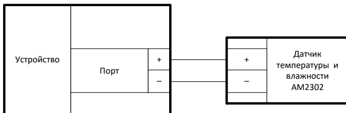
Рисунок 18 – Схема подключения датчика температуры и влажности
