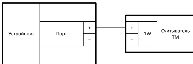
Рисунок 15 – Схема подключения считывателя ключей
