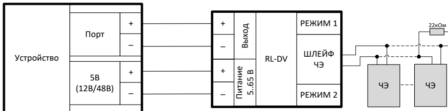
Рисунок 17 – Подключение шлейфа затопления через RL-DV
