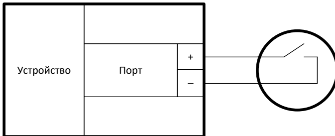
Рисунок 7 – Подключение датчика с выходом типа «Сухой контакт»
