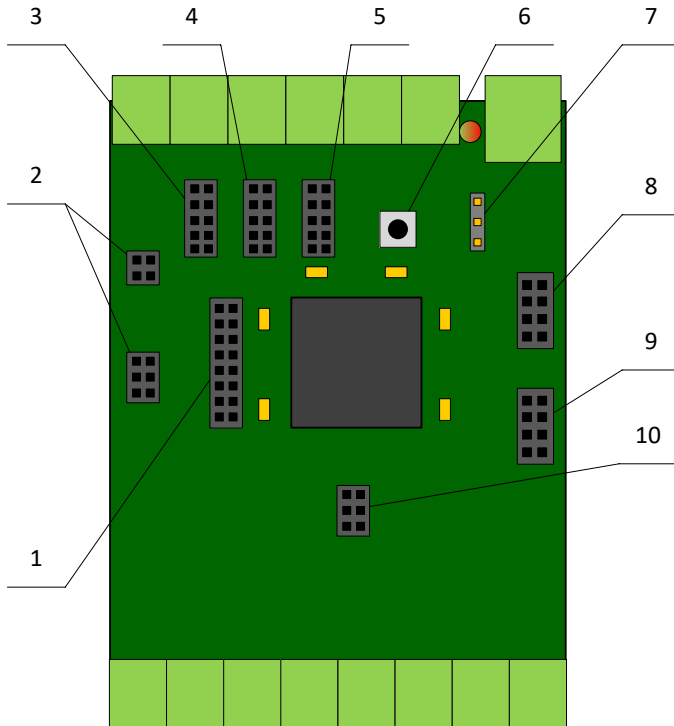
Рисунок 3 – Расположение элементов на плате Устройства
