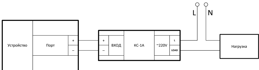
Рисунок 12 – Подключение симисторного ключа
