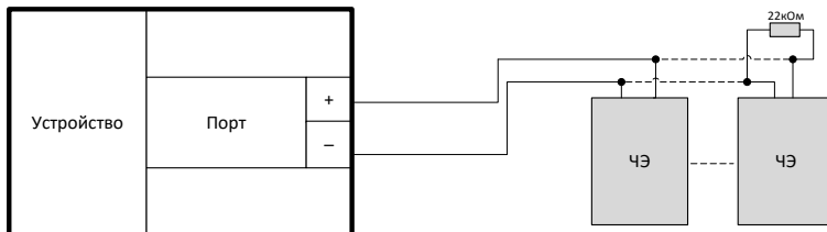
Рисунок 16 – Подключение шлейфа затопления
