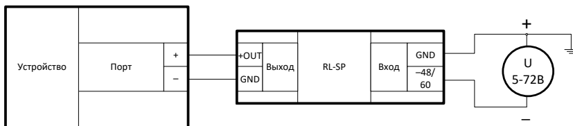
Рисунок 10 – Подключение модуля RL-SP для измерения напряжения
