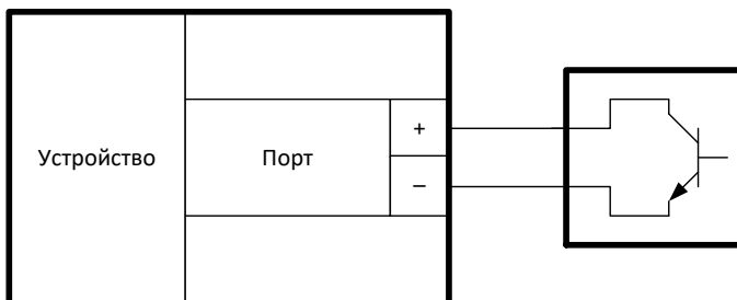
Рисунок 9 – Подключение датчика с выходом типа «Открытый коллектор»
