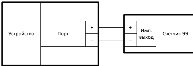
Рисунок 11 – Подключение импульсного выхода счетчика электроэнергии
