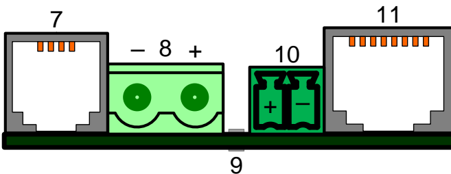
Рисунок 4 – Сторона интерфейсов и питания
