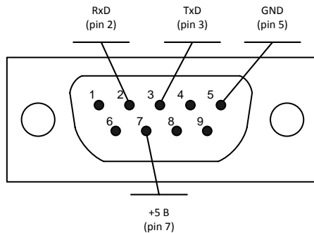
Рисунок 19 – Распиновка разъема DB9 для желтого(белого) кабеля
