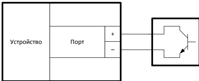
Рисунок 7 – Подключение датчика с выходом типа «Открытый коллектор»
