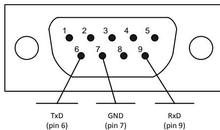
Рисунок 20 – Распиновка разъема DB9 для черного кабеля
