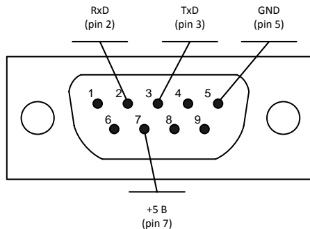
Рисунок 19 – Распиновка разъема DB9 для желтого(белого) кабеля
