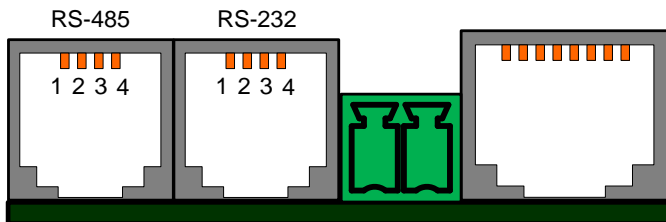
Рисунок 18 – Разъемы последовательных интерфейсов
