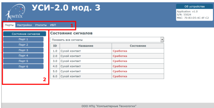
Рисунок 2 – Веб-страница Устройства
