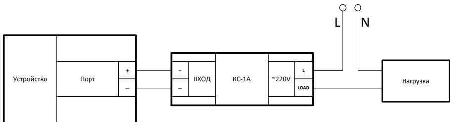
Рисунок 11 – Подключение симисторного ключа
