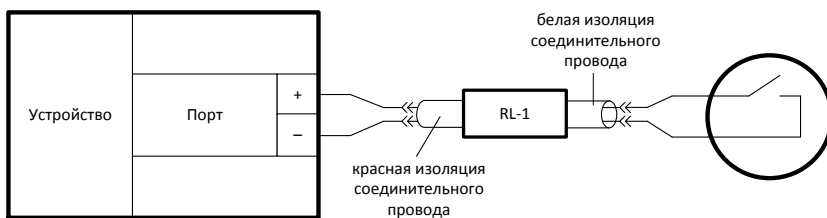
Рисунок 7 – Подключение датчика с помощью модуля RL-1
