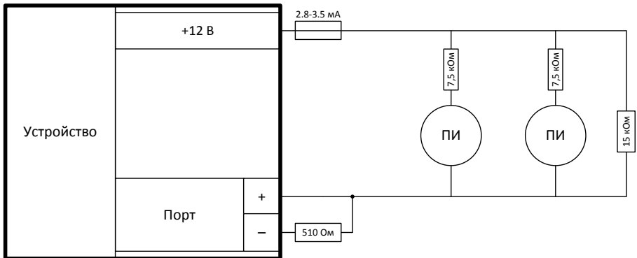
Рисунок 18 – Схема подключения пожарного шлейфа
