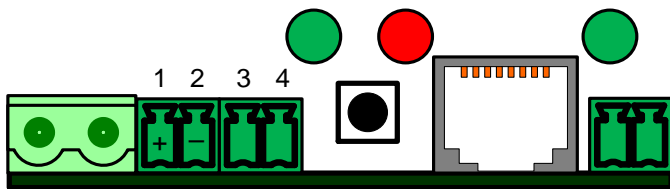
Рисунок 19 – Разъем последовательного интерфейса
